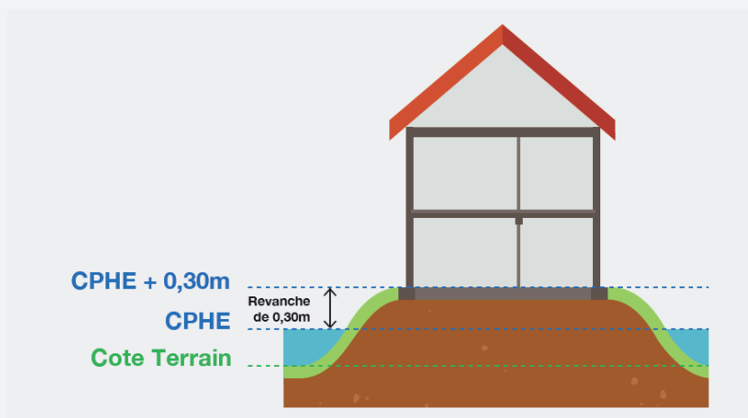
Figure 7 : Illustration de l'implantation d'un bâtiment en zone de débordement de cours d'eau. Source : Mayane pour la DDT du Bas-Rhin, 2018.
