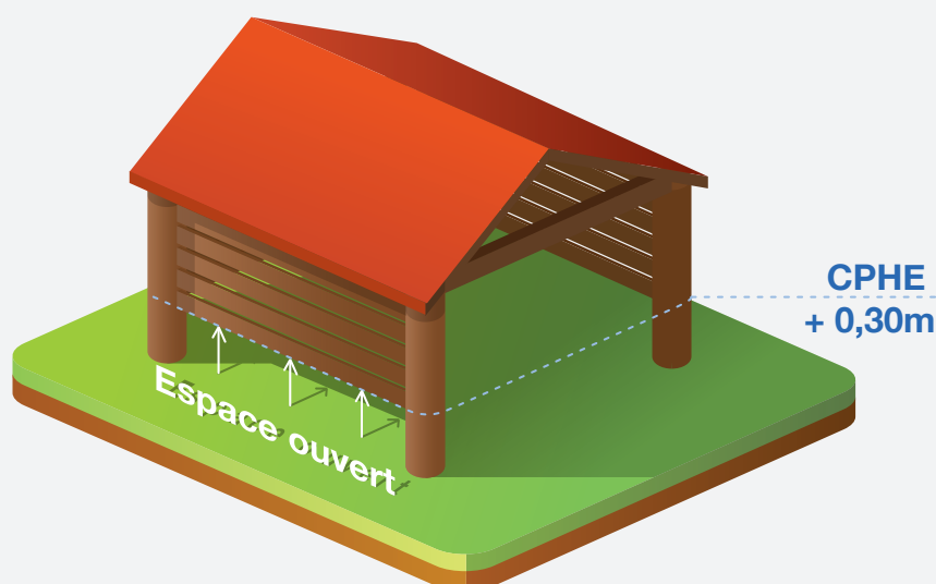
Figure 5 : Illustration d'un bâtiment ne comportant pas de paroi sous la CPHE. Source : Mayane pour la DDT du Bas-Rhin, 2017.
